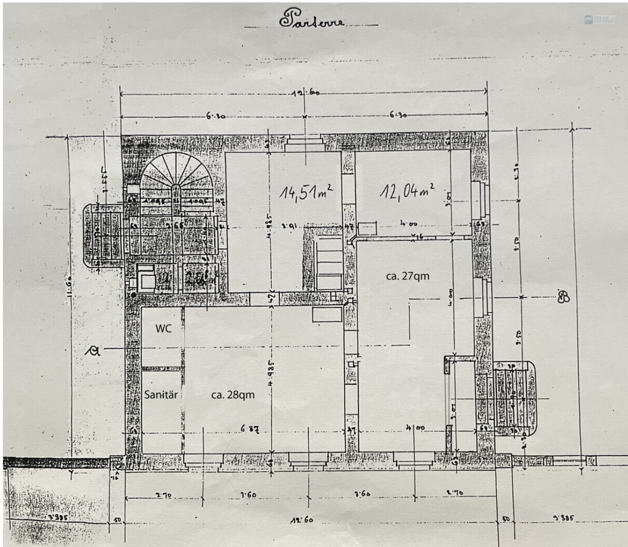
Grundriss
