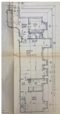
Grundriss
